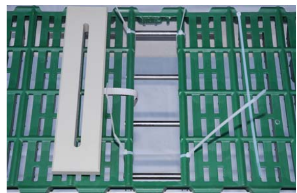
8. Mit 4 Kabelbindern fixierte Kassette
