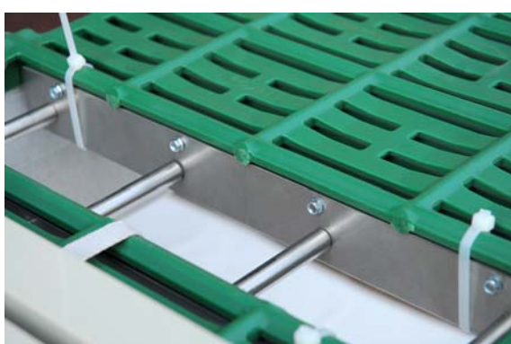
12. vollständig verschraubte Kassette. Kabelbinder entfernen.
