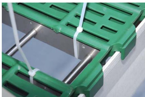
7. Kassette mit Kabelbindern fixieren
