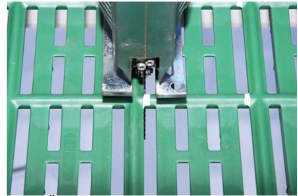
2. Öffnung stegbündig ausschneiden
